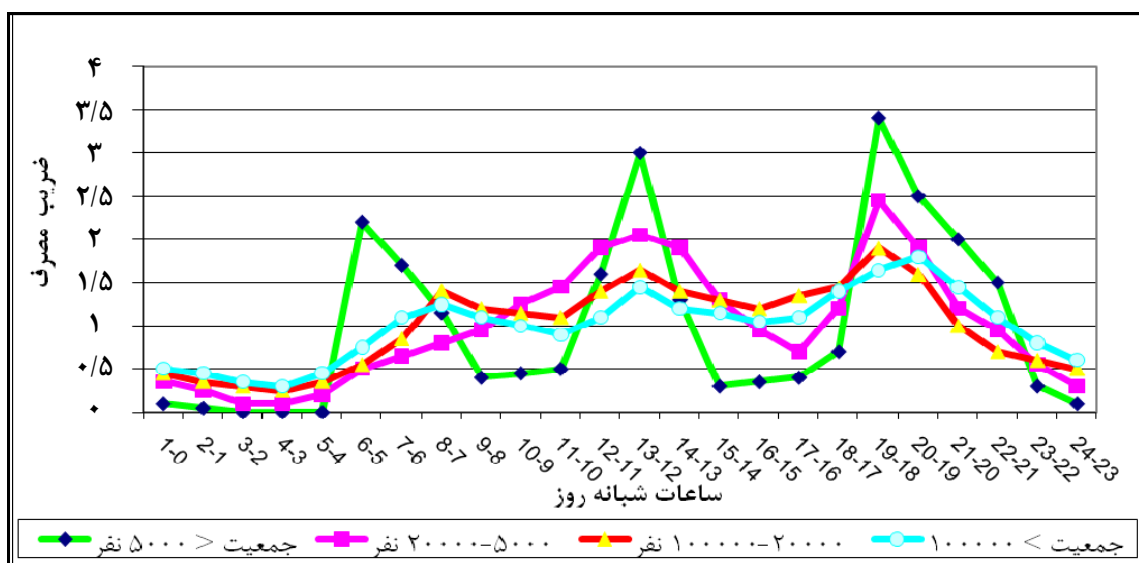
شکل ۳-۱- نمونه‌ای از نوسانات ساعتی مصرف
