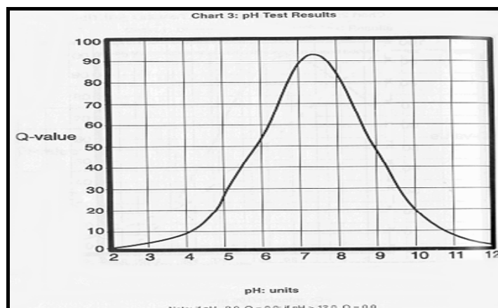
شکل پ.۵-۶- نمودار تعیین کیفیت آب بر اساس پارامتر PH
