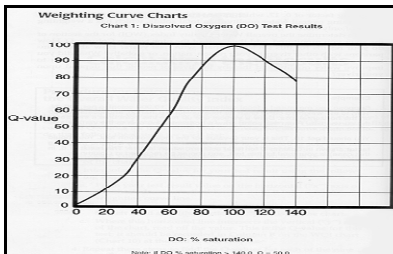
شکل پ.۵-۵- نمودار تعیین کیفیت آب بر اساس پارامتر اکسیژن محلول
