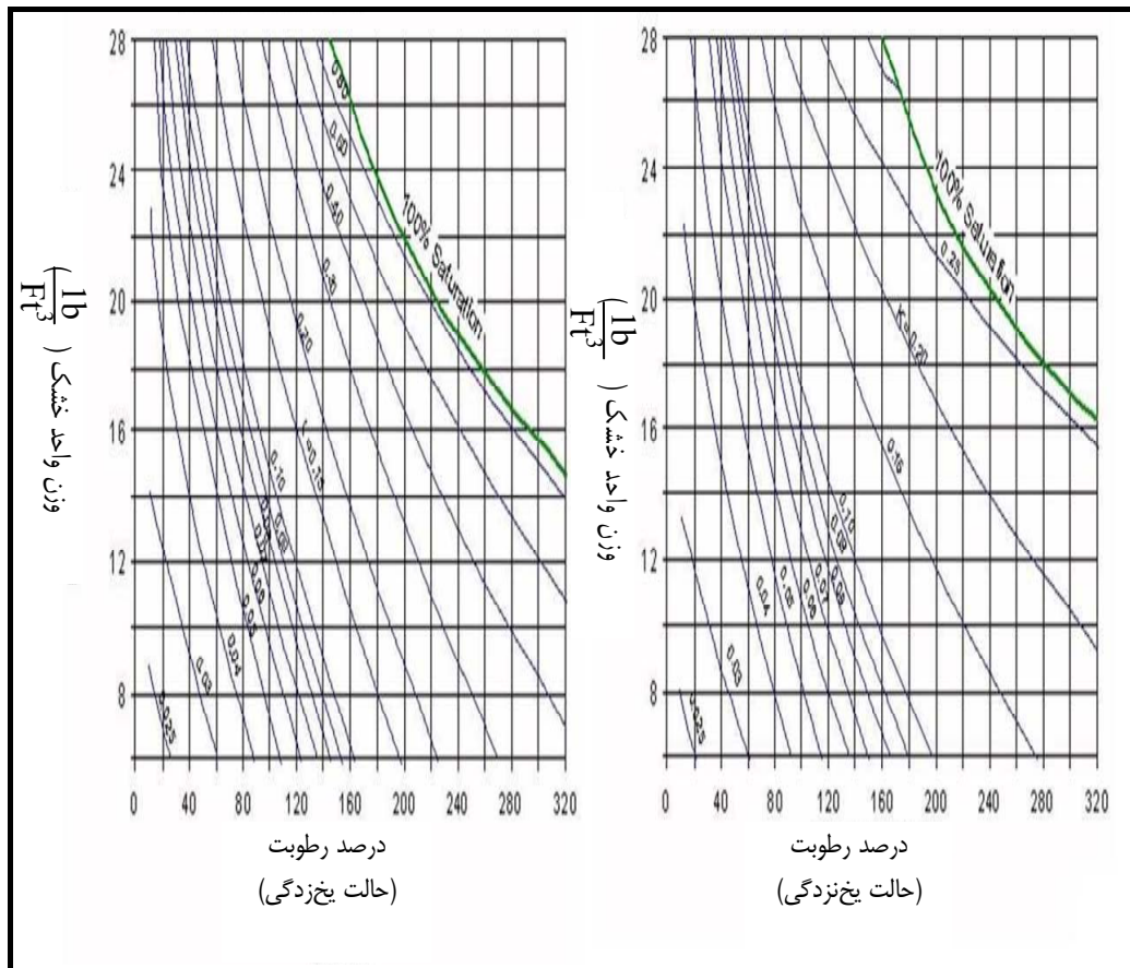
شکل پ. ۱-۶- متوسط ظرفیت انتقال حرارتی برای خاک‌های نباتی در دو حالت یخ‌زدگی و یخ‌نزدگی (برگرفته از Kersten, 1949 and Air Force, 1966)
