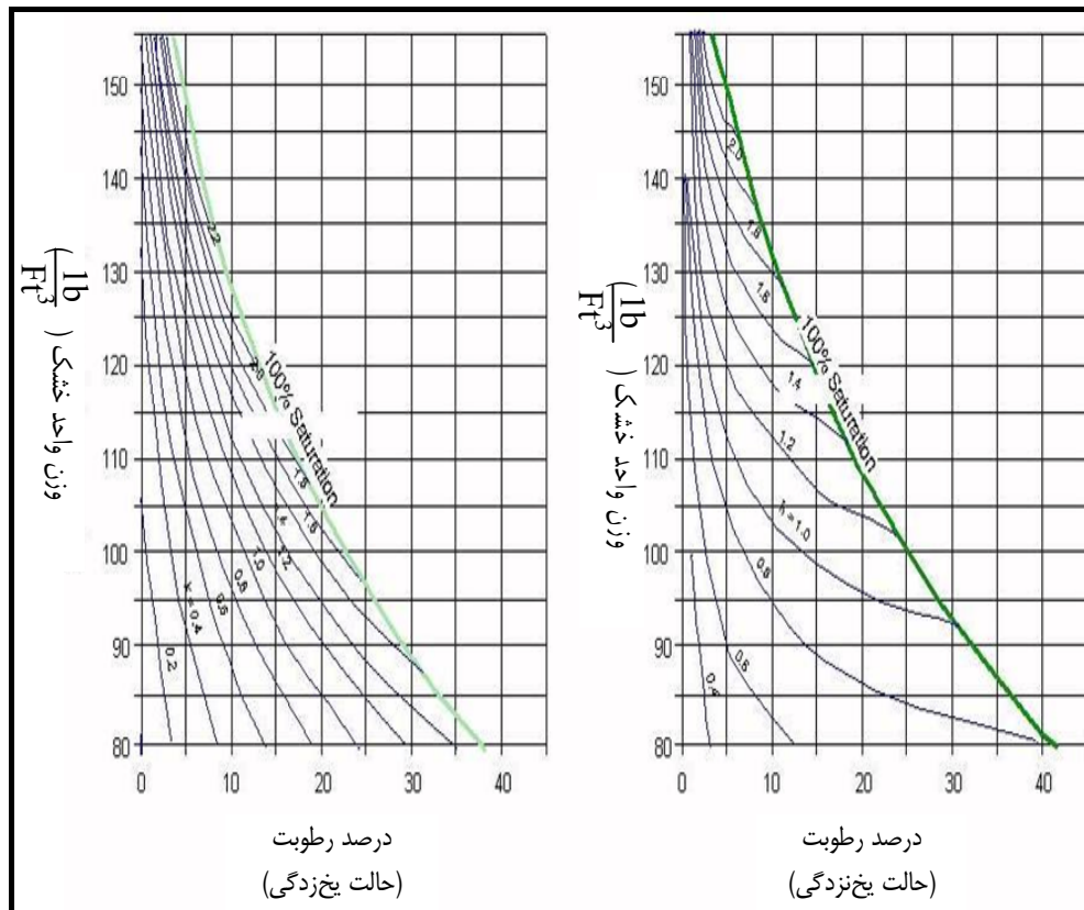
شکل پ. ۱-۵- متوسط ظرفیت انتقال حرارتی برای خاک‌های گرانولی در دو حالت یخ‌زدگی و یخ‌نزدگی (برگرفته از Kersten, 1949 and Air Force, 1966)
