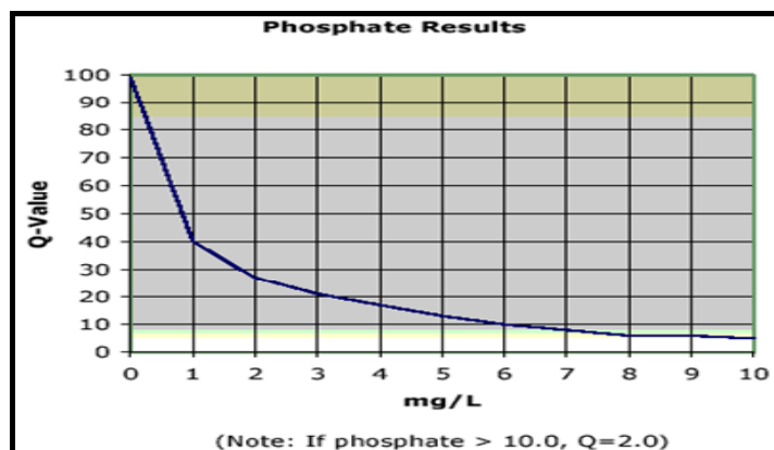
شکل پ.۵-۲- نمودار تعیین کیفیت آب بر اساس پارامتر فسفات
