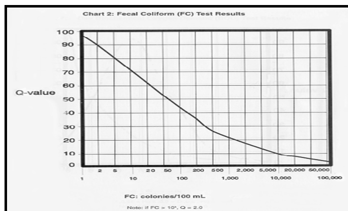
شکل پ.۵-۳- نمودار تعیین کیفیت آب بر اساس پارامتر فیکال کلیفرم
