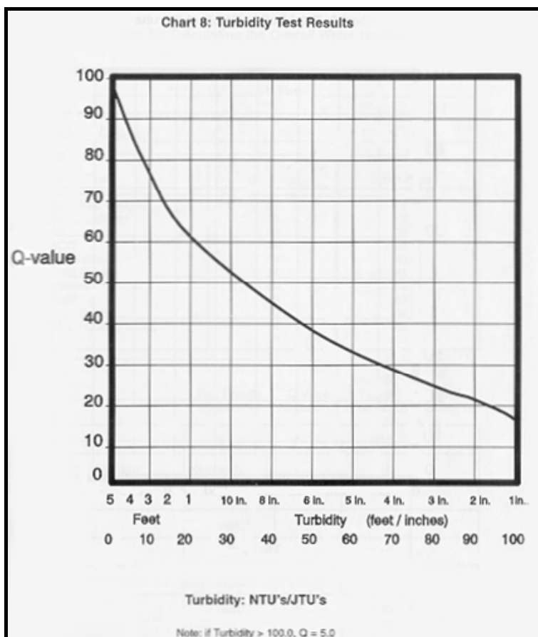
شکل پ.۵-۴- نمودار تعیین کیفیت آب بر اساس پارامتر کدورت
