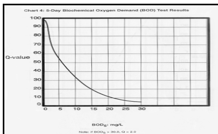
شکل پ.۵-۸- نمودار تعیین کیفیت آب بر اساس کل B.O.D
